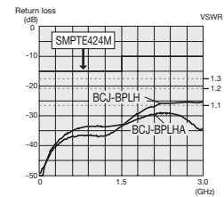
Return loss for BCJ-BPLHA, BCJ-BPLH
