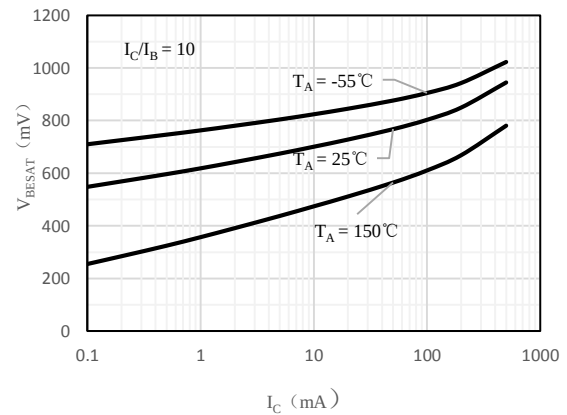
Fig 6 V_{BE(sat)} vs. I_C
