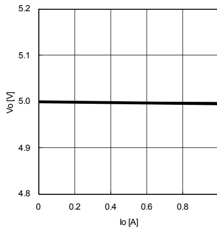
Fig.11 Io-Vo
