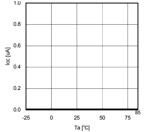
Fig.9 Ta-I sd
