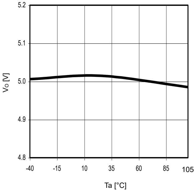
Fig. 21 Ta-V_O ( I_O=0mA )
