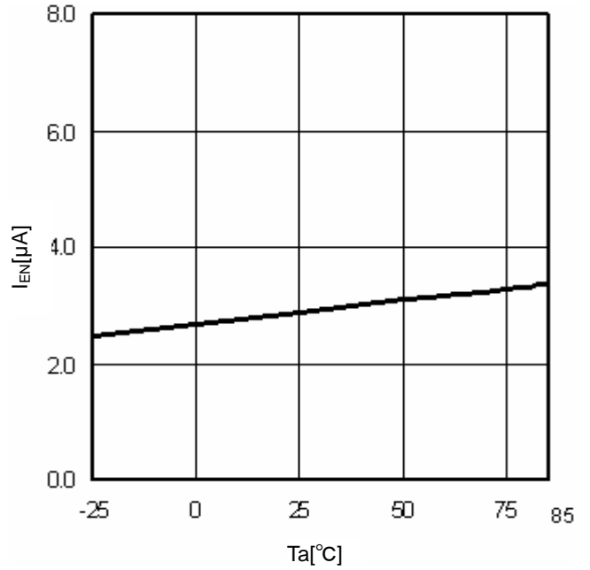
Fig.11 T_a - I_{EN}
