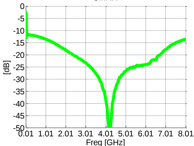
CMRR
