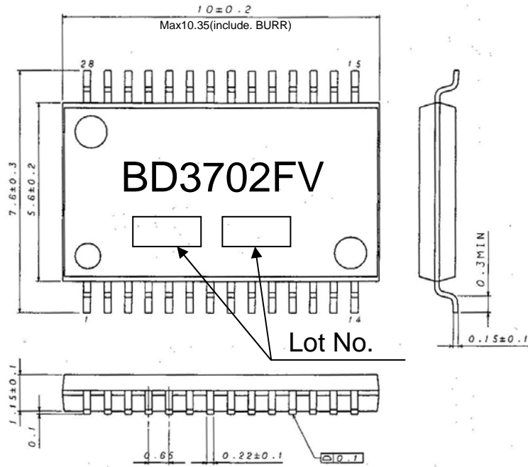
SSOP-B28 (Unit : mm)
