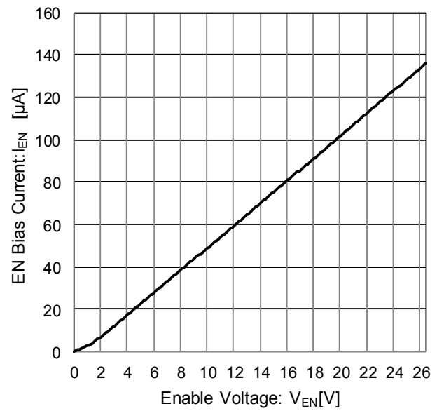
Figure 44. EN Voltage vs EN Current
