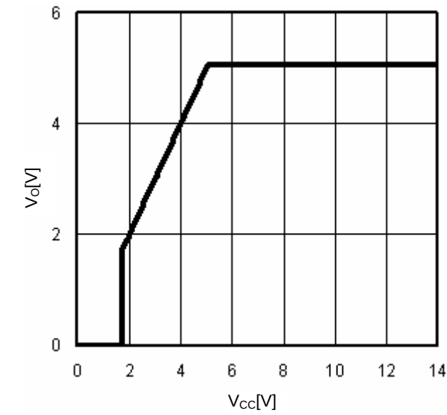
Fig.15 V CC -V O (I O =0mA)
