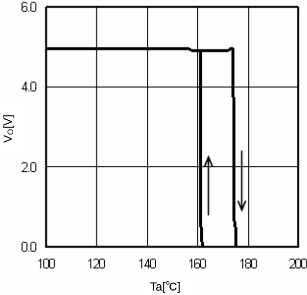
Fig.16 TSD (I O =0mA)
