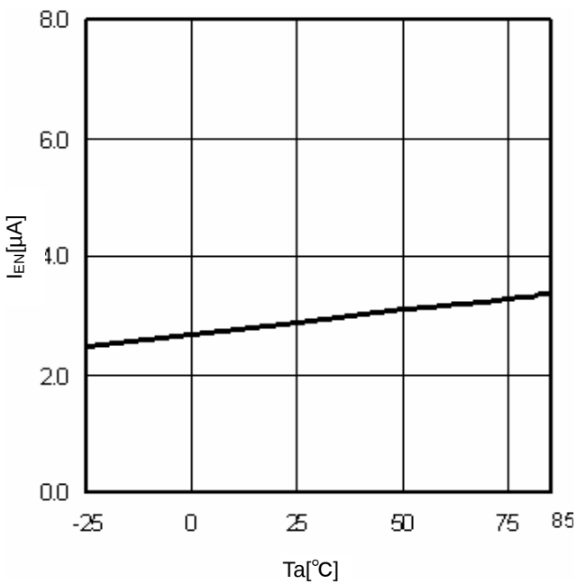
Fig.12 T_a - I_{EN}
