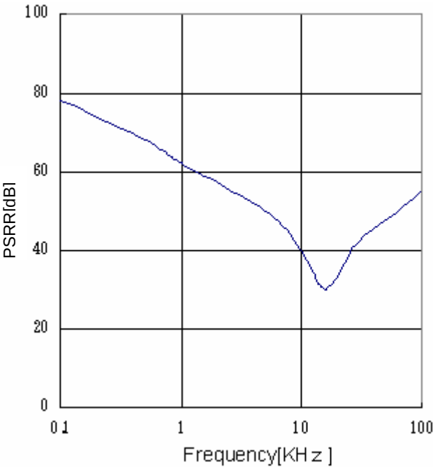
Fig.21 PSRR ( I_o=0 mA)
