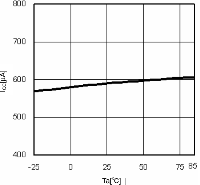
Fig.10 T_a - I_{cc}
