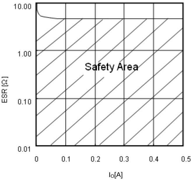
Fig.19 ESR condenser
