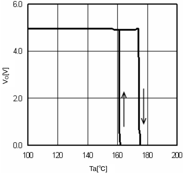
Fig.16 TSD ( I_o=0mA )
