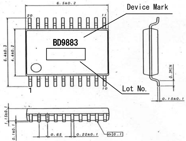
SSOP-B20 (Unit:mm)
