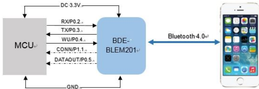
图 2.1 模块与手机连接通信
