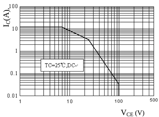
SOA
