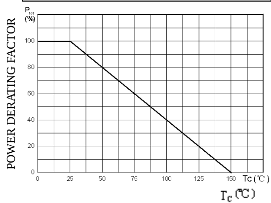
P_C - T_C
