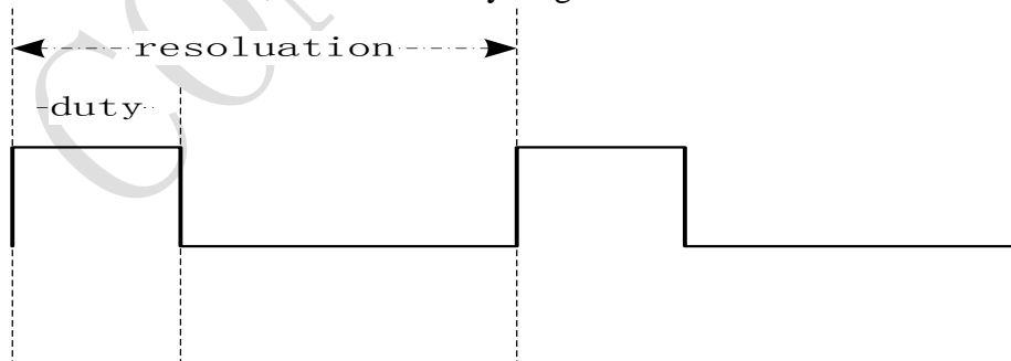
Figure 15 PWM parameter
