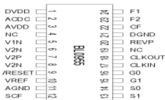
SSOP24
