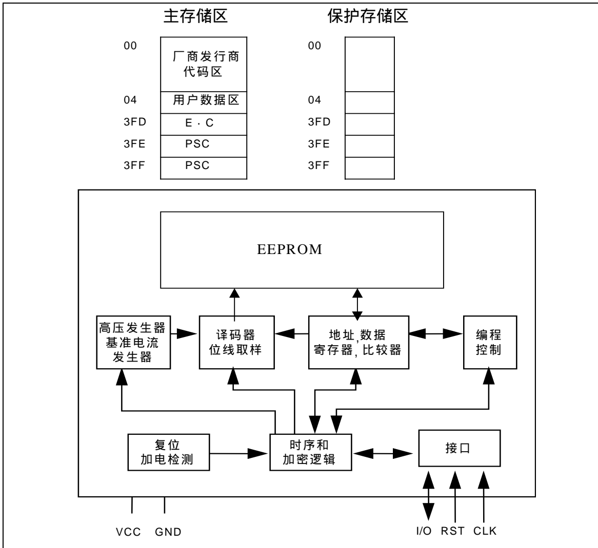
图 2 电路框图和存储空间分布
