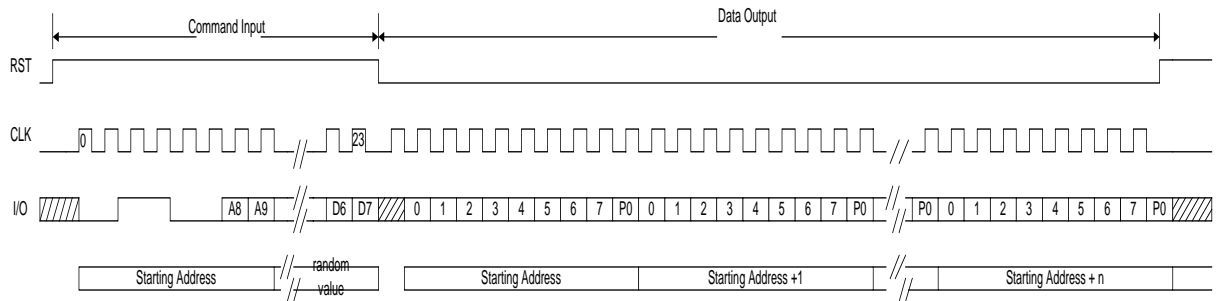
图 8 读数据字节包括保护位时序图
