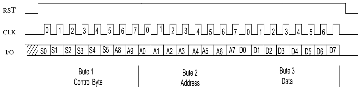
图4 命令输入时序图
