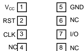
图 1 管脚图
