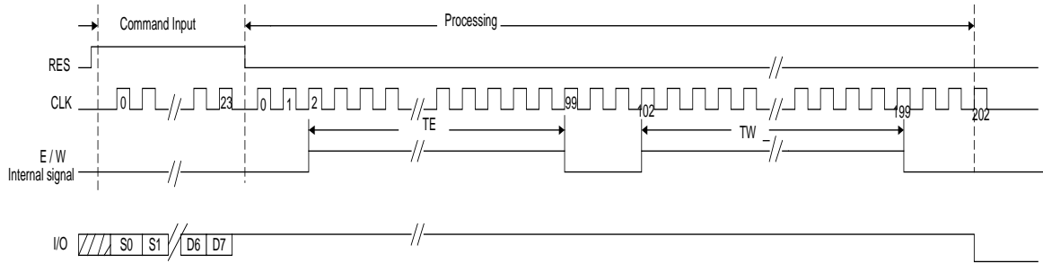
图 5 擦除并写入时序图
