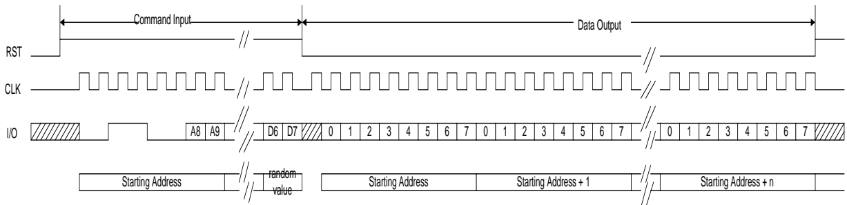
图 7 读数据字节时序图
