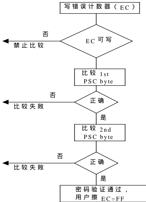
图 9 密码验证流程图
