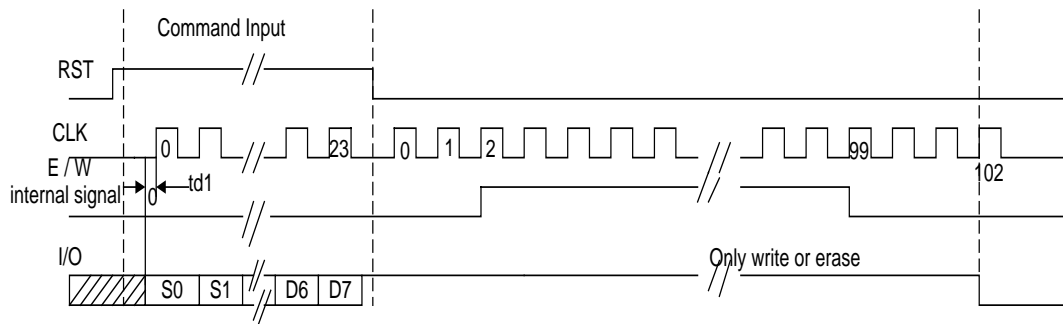
图 6 只写只擦时序图
