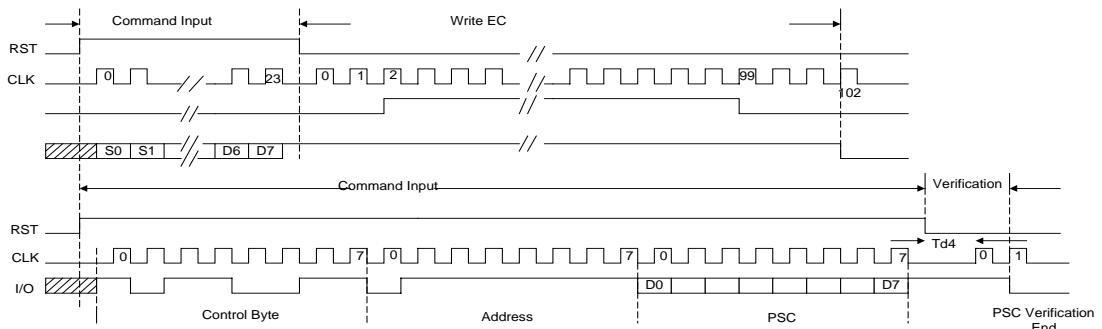
图 10 PSC 验证时序图
