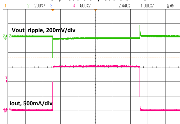
Ch2—Vout_ripple, Ch4—Iout
