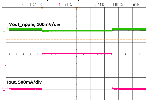
Ch2—Vout_ripple, Ch4—Iout
