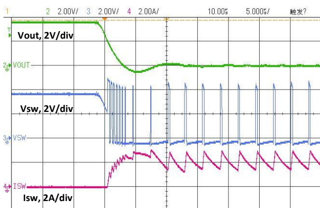
Ch2—Vout, Ch3—Vsw, Ch4—Isw
