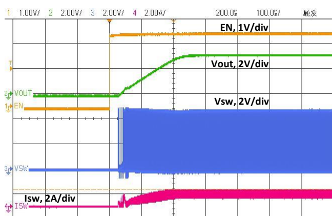
Ch1—EN, Ch2—Vout, Ch3—Vsw, Ch4—Isw
