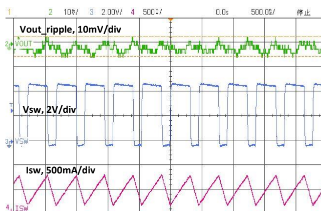
Ch2—Vout_ripple, Ch3—Vsw, Ch4—Isw
