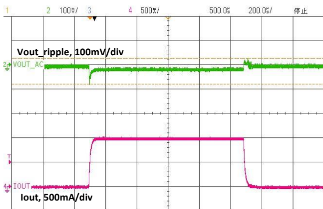
Ch2—Vout_ripple, Ch4—Iout
