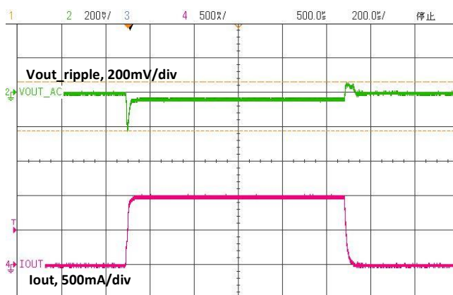
Ch2—Vout_ripple, Ch4—Iout
