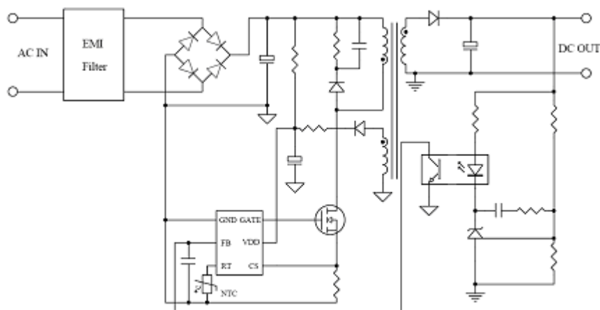
图 1. 典型应用图
