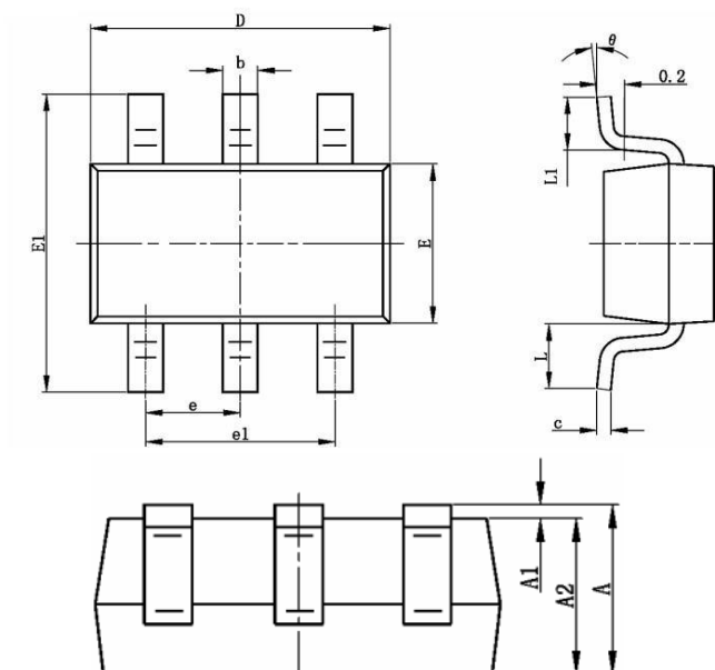
SOT-23-6 封装尺寸
