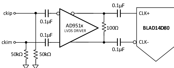
图 35. 差分LVDS采样时钟(频率可达625 MHz)
