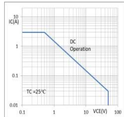
SOA
