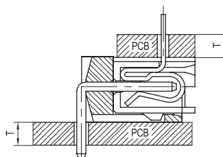
PCB ASS'Y
