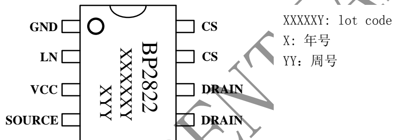
图 2 管脚封装图
