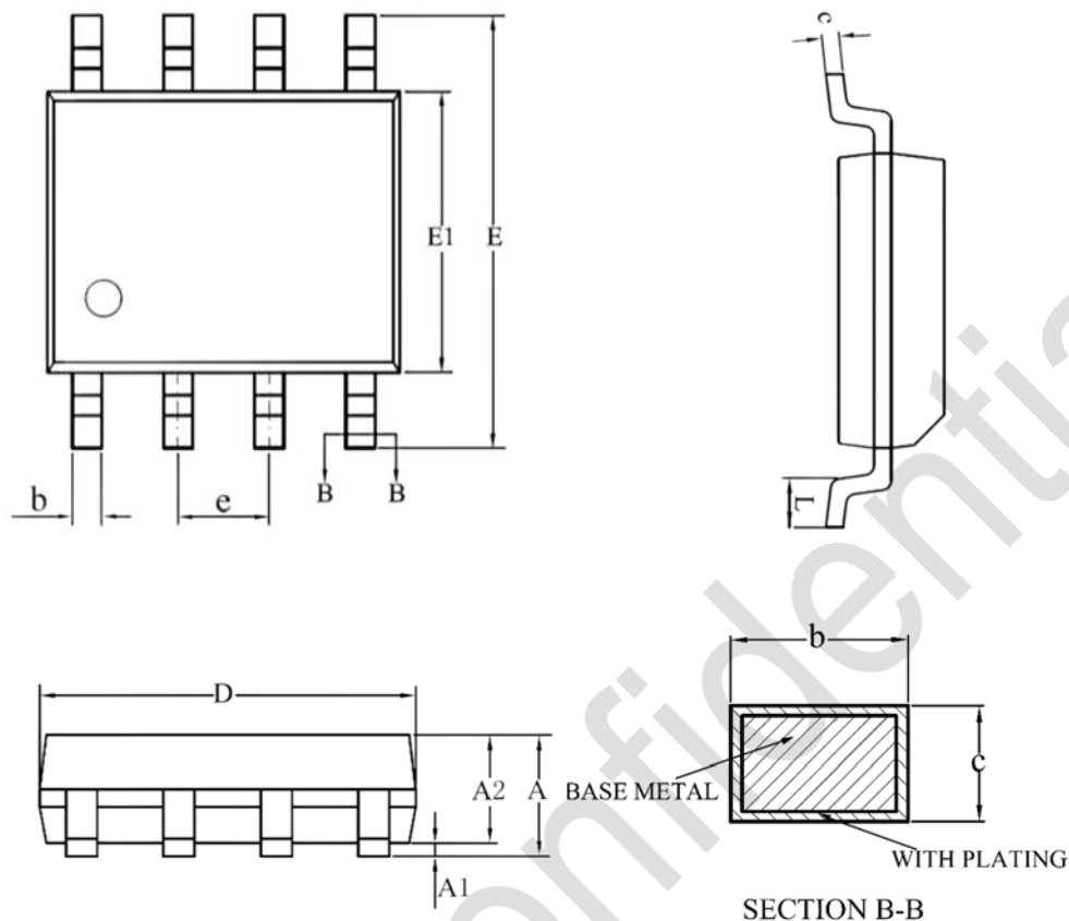
SOP-8 封装外形尺寸
