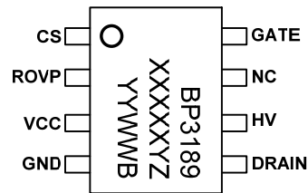
图 2 管脚封装图
