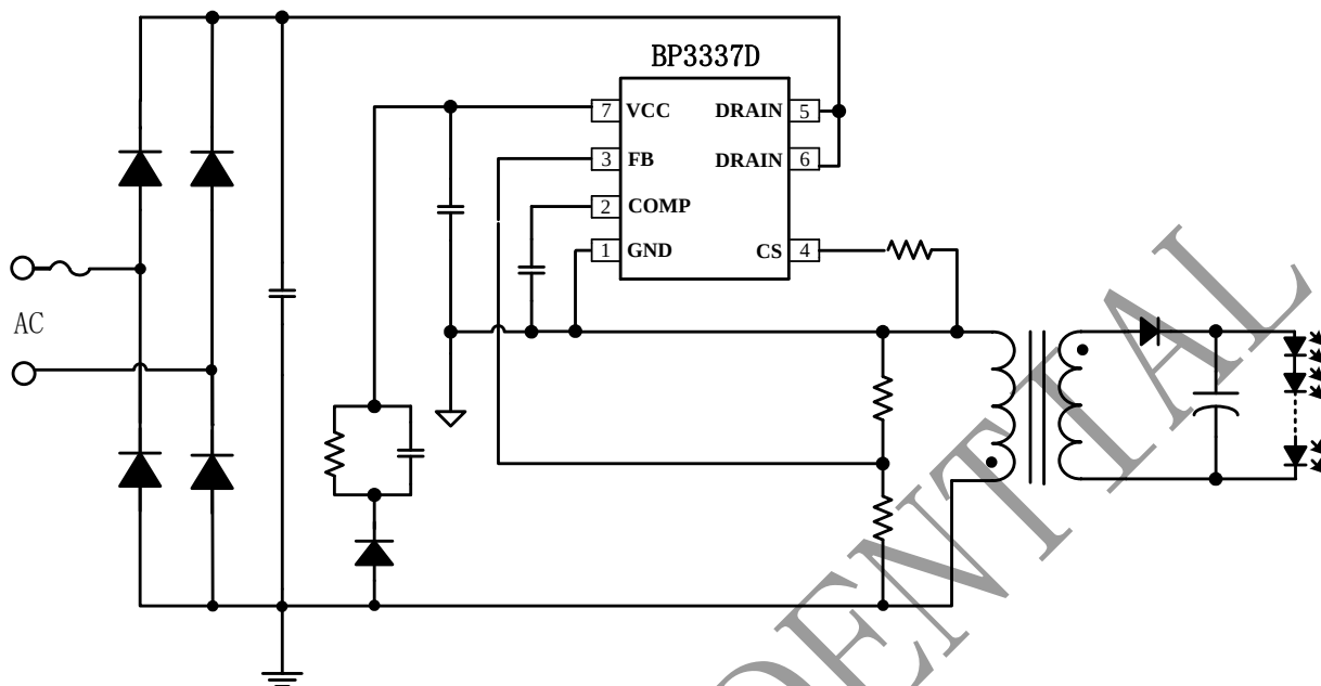
图 1 BP3337D 浮地双绕组隔离反激典型应用图
