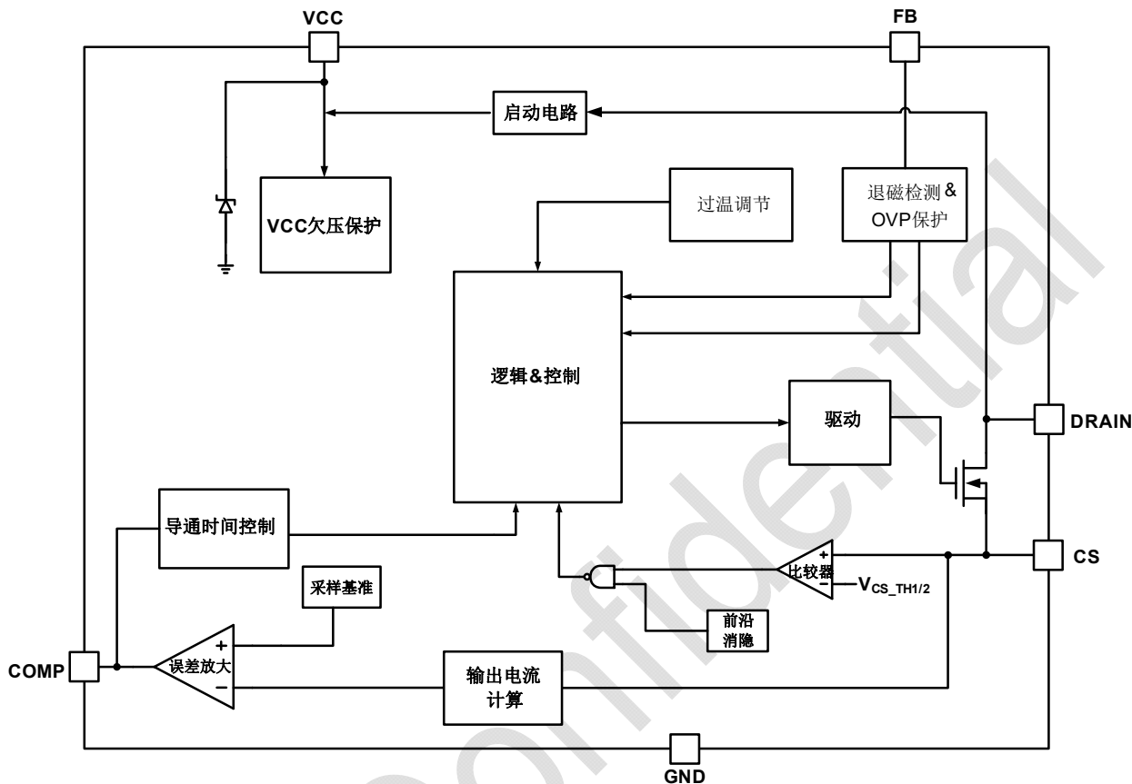
图 3 BP3337EB 内部框图
