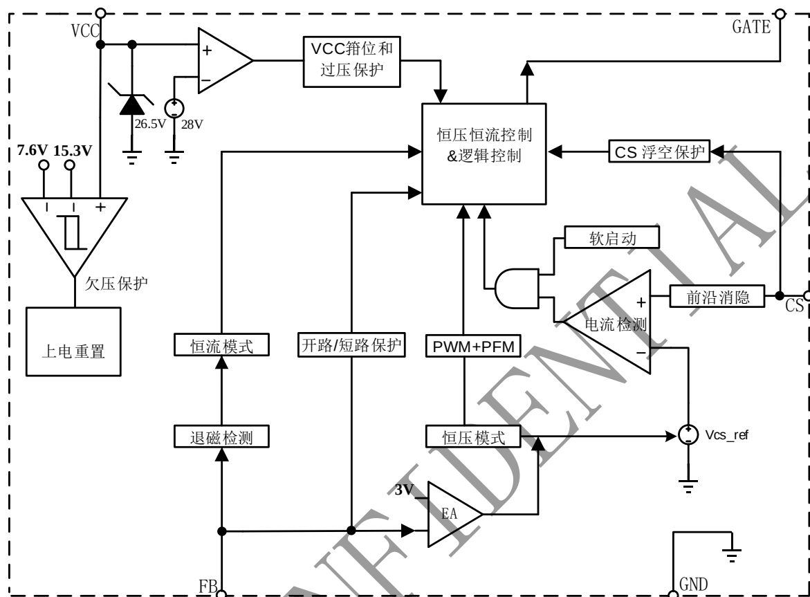
图 3 BP6519 内部框图
