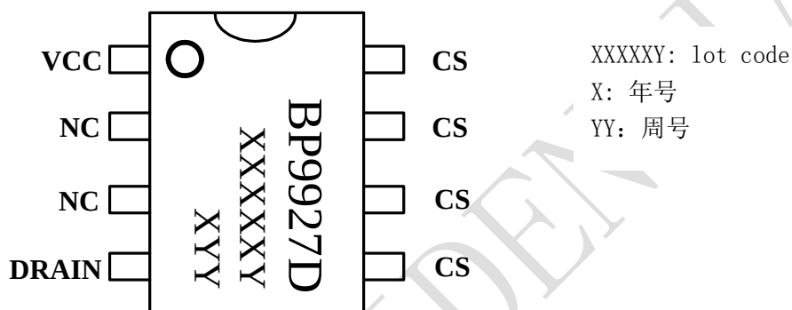
图 2 管脚封装图
