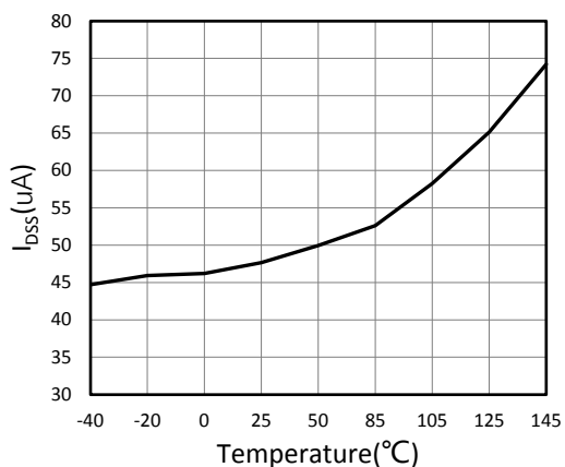
图 14. I DSS vs. Temperature
