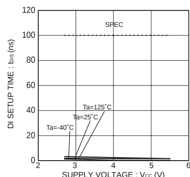
Fig.19 DI setup time t_{DIS}
