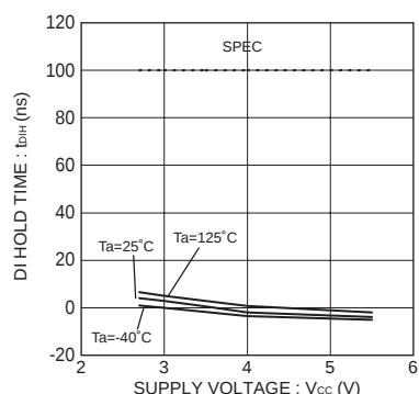
Fig.20 DI hold time t_{DIH}
