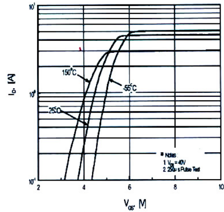
I_D - V_{GS}
