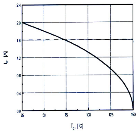
I_D - T_c
