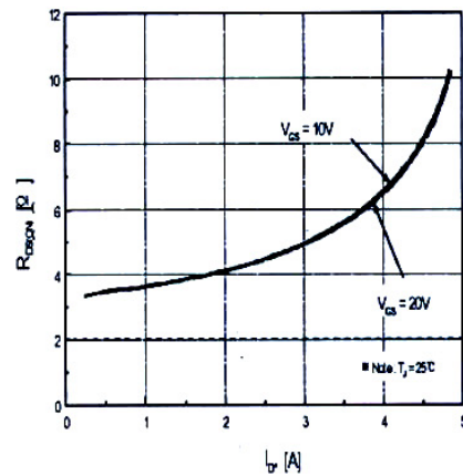
R_{DS(on)} - I_D
