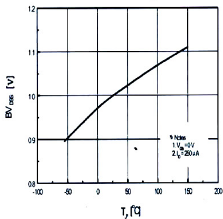
BV_{DSS} - T_J
