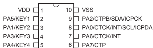
BS83B04C 10 DFN-A
