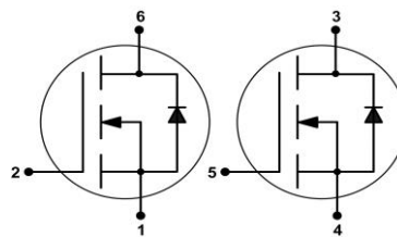
PG-SOT-363
