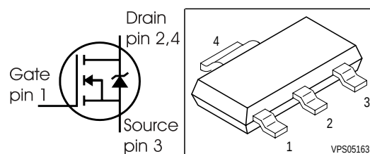
SOT-223
