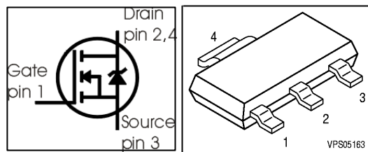
SOT-223
