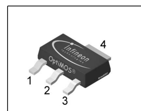
SOT 223
