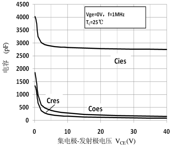
图 7. 电容特性
