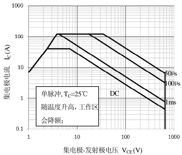
图 12. 安全工作区
