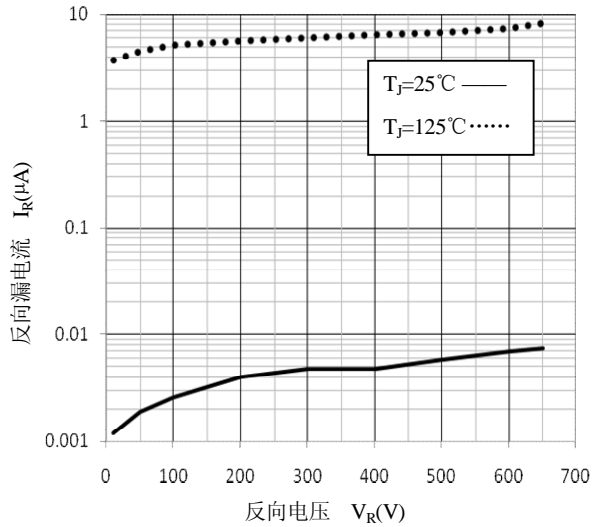
图 16. 二极管反向漏电流特性
