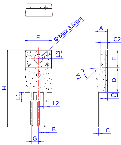
TO-220F Ins
