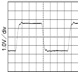
Fig.21 VCXO_OUT(27MHz) output waveform VDD=3.3V,CL=4pF
