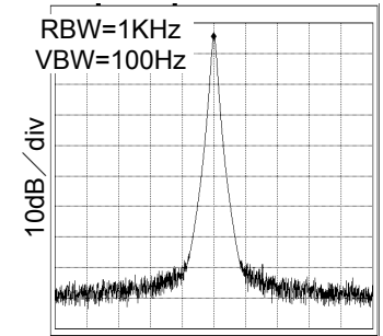
Fig.23 VCXO_OUT(27MHz) spectrum VDD=3.3V,CL=4pF
