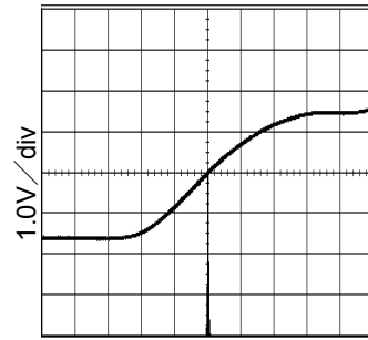
Fig.22 VCXO_OUT(27MHz) Period-Jitter VDD=3.3V,CL=4pF
