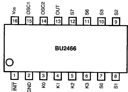
BU2466 pin layout
