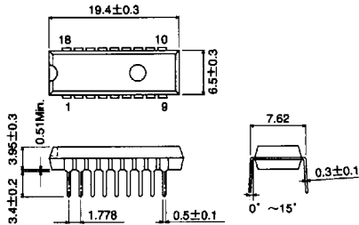
SDIP18
