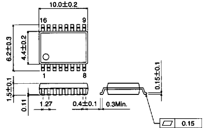
SOP16
