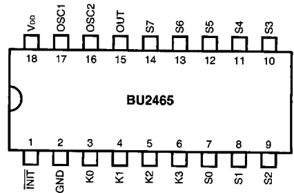
BU2465 pin layout
