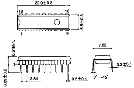
DIP18
