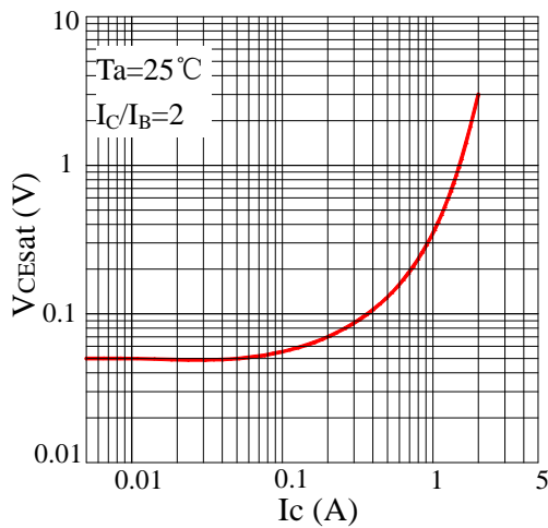
Fig5 V CEsat -I C
