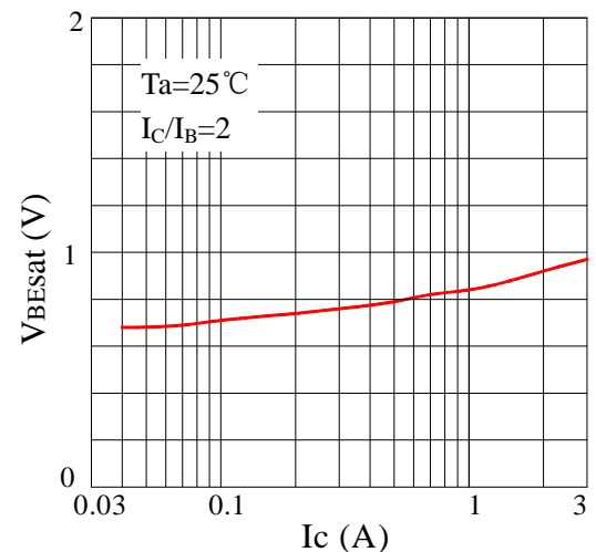
Fig6 VBEsat-Ic
