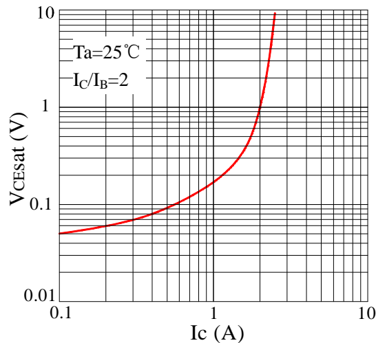
Fig5 VCESat-Ic
