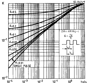
Thermal impedance
