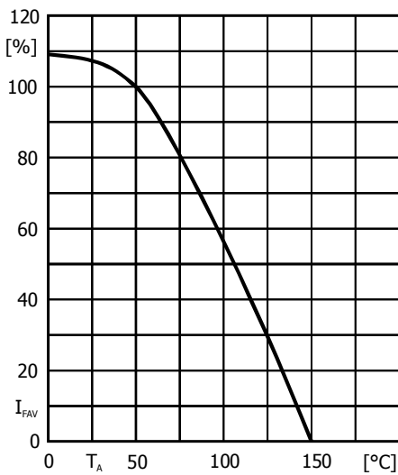
Rated forward current versus ambient temperature Zul. Richtstrom in Abh. von der Umgebungstemp.
