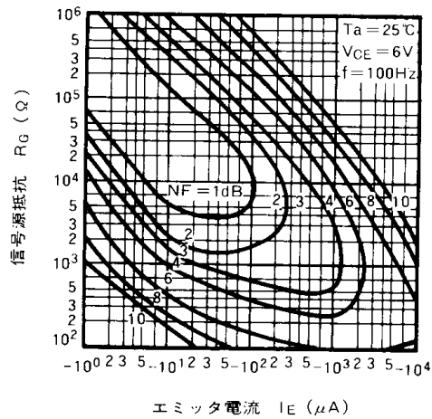
雑音指数特性 ( f=100\text{Hz} )
