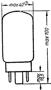
max. Abmessungen
