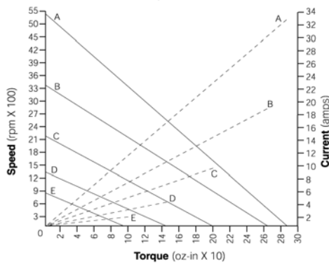
C23-L55: 36 Volt input
