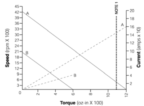
C34-L80: 24 Volt input
