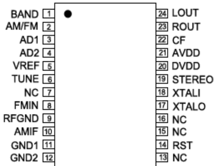
(表 7. CA9610 芯片引脚描述)
