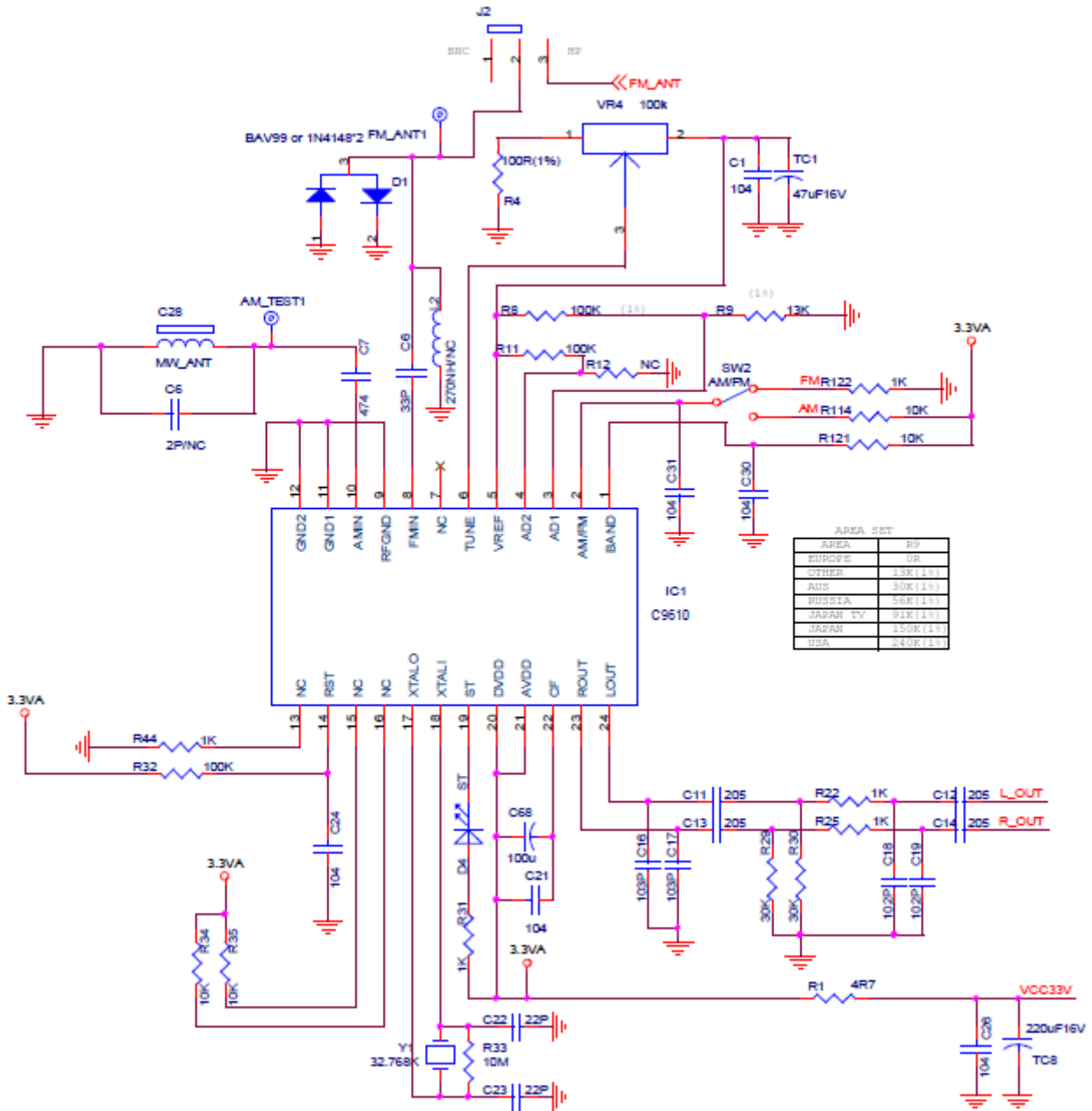
(图 11. 典型应用原理图)
