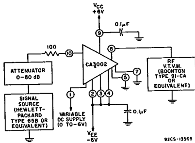
Fig. 18 - AGC range.
