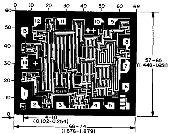
CD4025B
