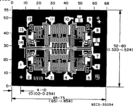
CD4001B
